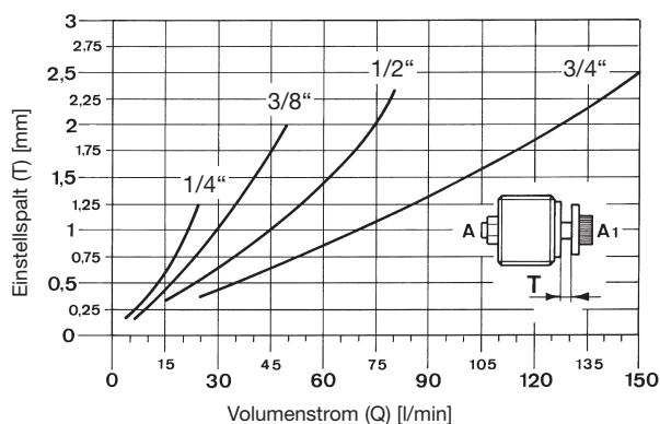
Einstelltabelle für Schließstrom
